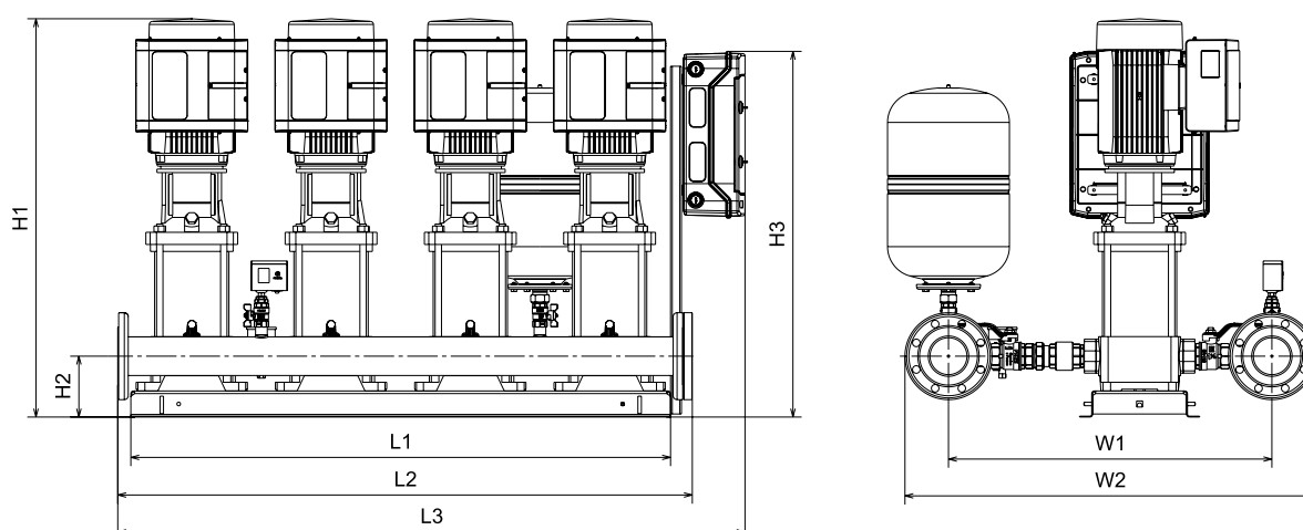
HC-ME 4 BME 10..64 (до 7,5 кВт)
